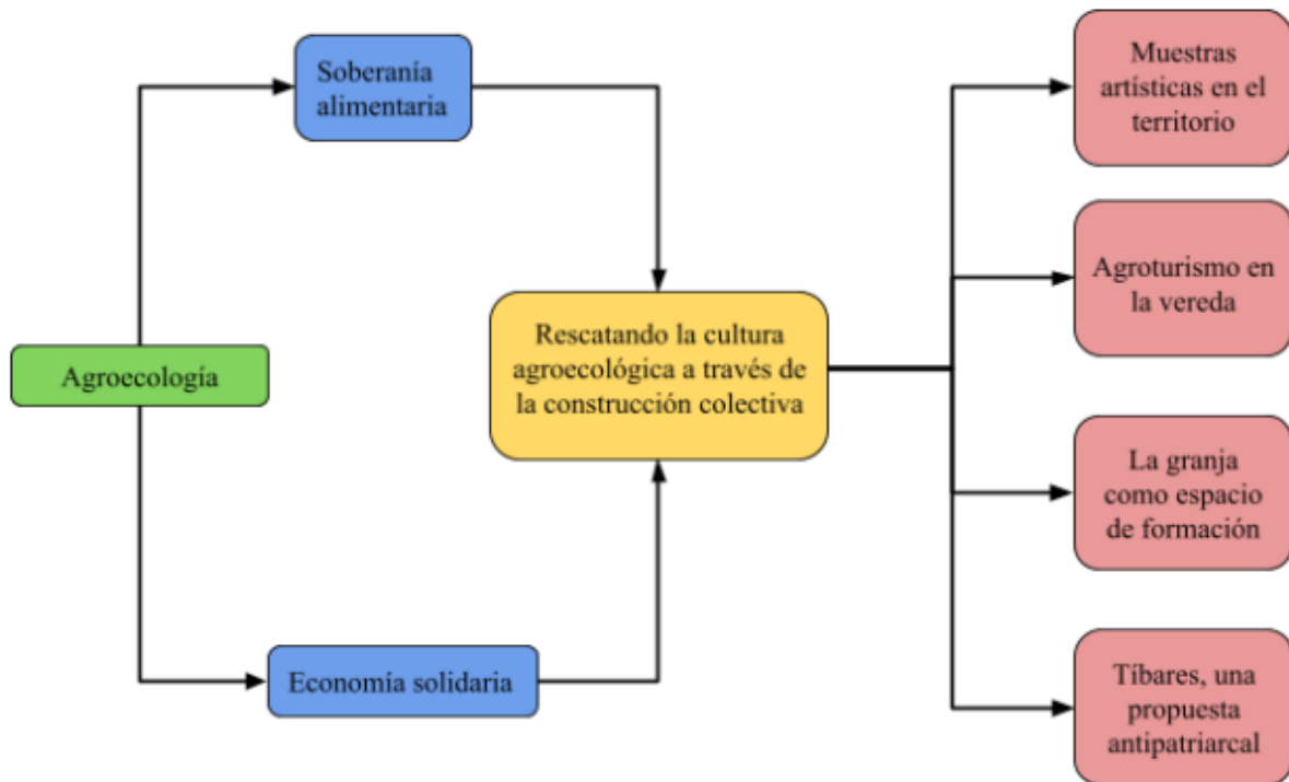
Figura 7. Taxonomía 1.
